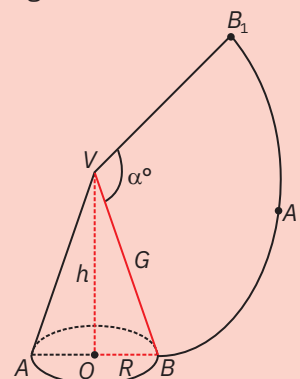
Figura 1. Conul circular drept și desfășurarea sa
