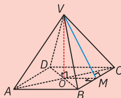
Figura 2 Piramidă patrulateră regulată
