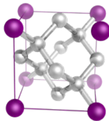
Structura diamantului
