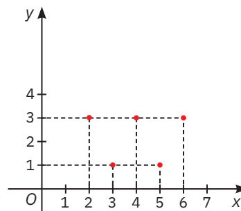
Figura 7: Graficul funcției g(n) = u(4^n) - 3
