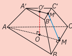
Figura 1 Trunchi de piramidă triunghiulară regulată
