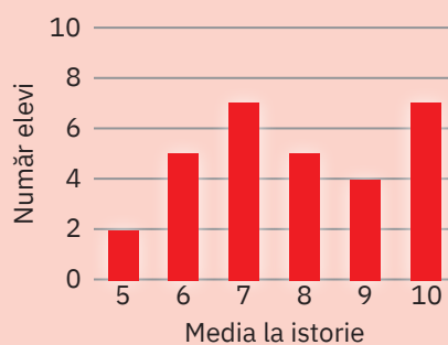
Date bimodale, cu modurile 7 și 10
