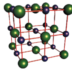
Structura sării de bucătărie
