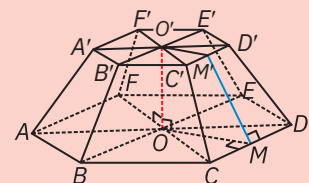
Figura 3 Trunchi de piramidă hexagonală regulată
