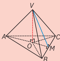
Figura 1 Piramidă triunghiulară regulată
