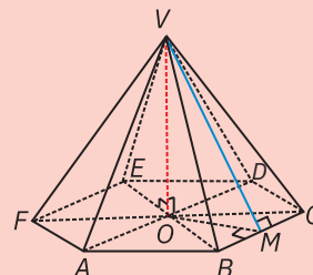
Figura 3 Piramidă hexagonală regulată
