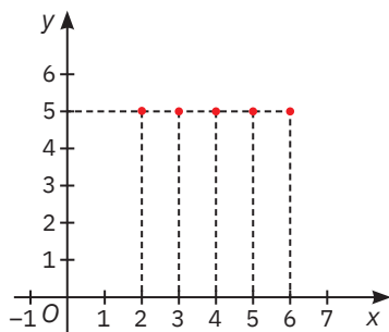
Figura 6: Graficul funcției f(n) = u(5^n)
