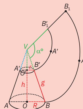
Figura 3. Trunchiul de con circular drept și desfășurarea sa
