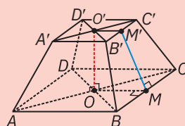
Figura 2 Trunchi de piramidă patrulateră regulată
