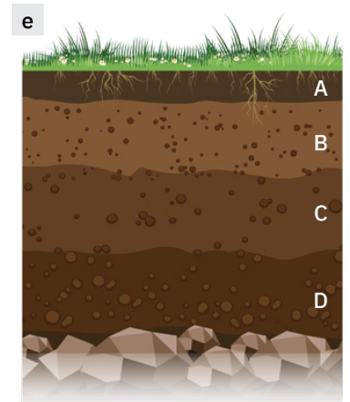
Profil de sol
