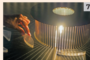
Lentilă planconcavă
