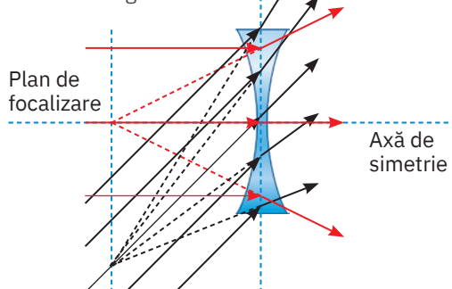
Lentilă divergentă
