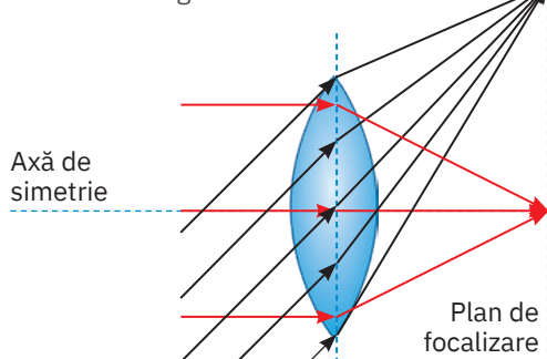
Lentilă convergentă
