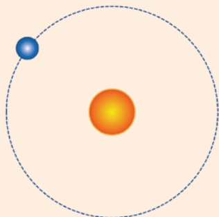
Un model atomic
