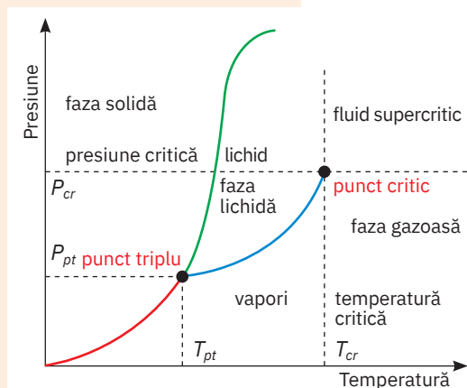
Diagrama de fază presiune-temperatură
