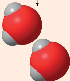
Apă
