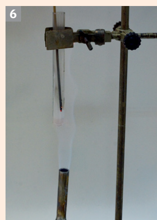
Introducerea așchii de lemn în eprubetă
