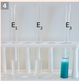
Solubilitatea \text{NaOH} , \text{KOH} , și \text{Cu}(\text{OH})_2 în apă
