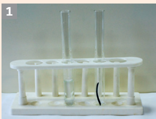
Eprubete cu soluție de acid sulfuric, respectiv panglică de magneziu
