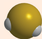
Molecula de acid sulfhidric, H 2 S
