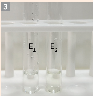
Soluții de bromură de potasiu, KBr, și iodură de potasiu, KI
