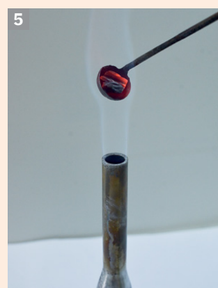
Arderea cărbunelui
