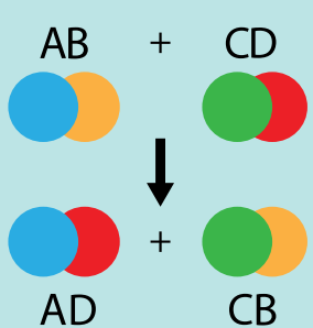
Reacția de schimb
