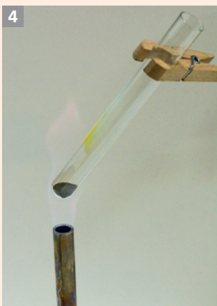
Reacția fierului cu sulf
