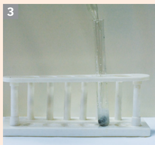
Reacția aluminiului cu acidul clorhidric
