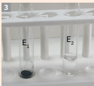
Oxid de cupru (II), \text{CuO} , și soluție de acid sulfuric, \text{H}_2\text{SO}_4
