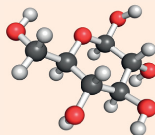
Molecula de glucoză, C_6H_{12}O_6
