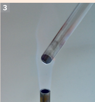
Obținerea mercurului din oxid de mercur
