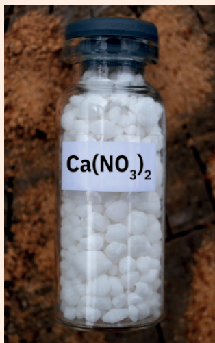
Azotat de calciu
