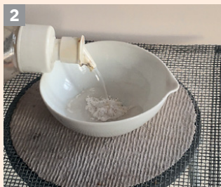
Adăugare de apă peste varul nestins
