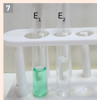
Soluție de sulfat de nichel (II), NiSO 4 , și soluție de hidroxid de sodiu, NaOH
