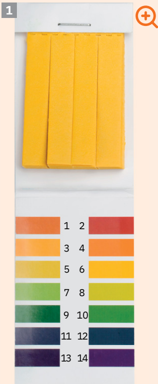
Hârtie de pH
