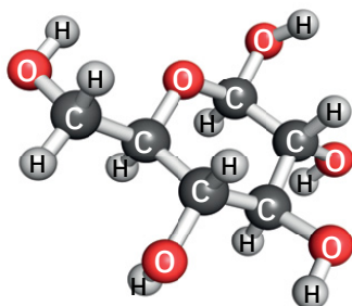
Molecula de glucoză
