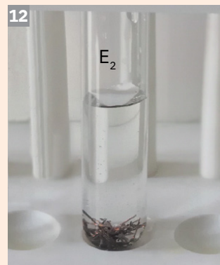
Cupru cu apă
