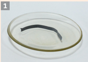
Panglică de magneziu
