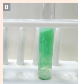
Obținerea hidroxidului de nichel (II), Ni(OH) 2
