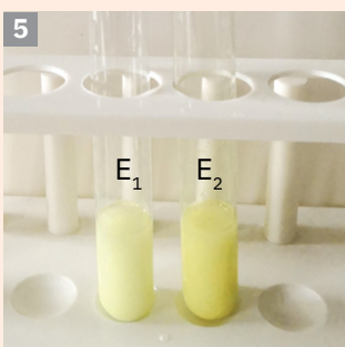
Formarea precipitatelor de bromură de argint, AgBr, și iodură de argint, AgI
