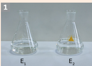
Paharele Erlenmeyer E 1 și E 2
