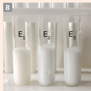
Formarea precipitatelor de sulfat de bariu, BaSO 4
