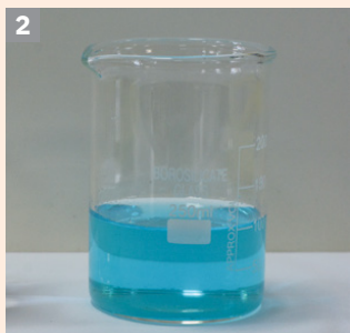
Soluție de sulfat de cupru, \text{CuSO}_4
