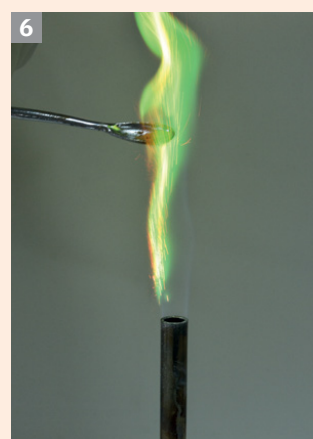
Arderea cuprului
