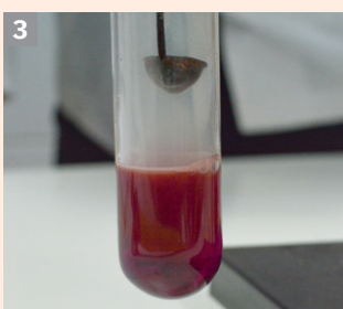
Înrșirea soluției de turnesol după arderea sulfului
