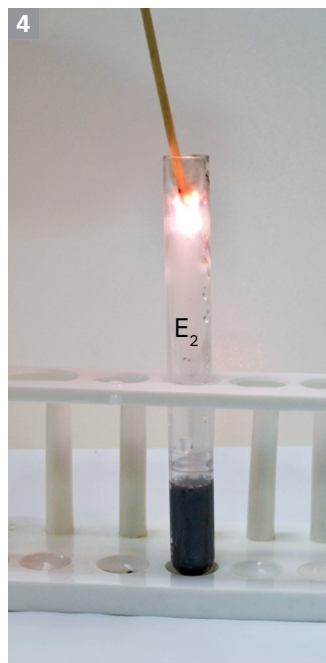
Eprubetele E_1 și E_2 cu apă oxigenată
