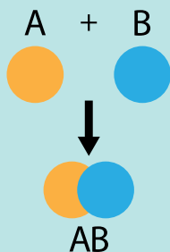
Reacția de combinare
