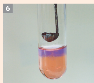
Înroșirea turnesolului
