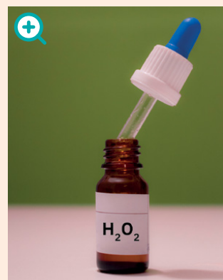
Apă oxigenată, H_2O_2
