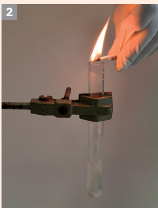
Arderea hidrogenului degajat din reacția magneziului cu acidul sulfuric
