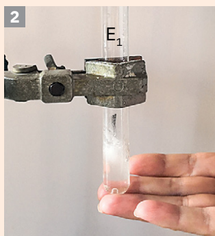
Reacția magneziului, Mg, cu acidul sulfuric, H_2SO_4
