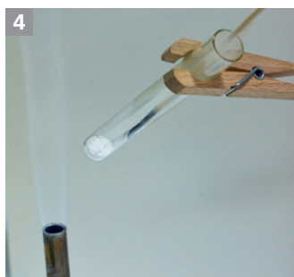
Introducerea unei așchii de lemn aprinsă în eprubetă
