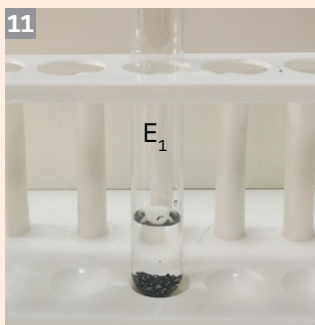
Magneziu cu apă
