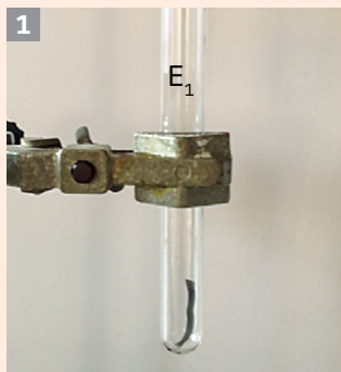
Panglică de magneziu
