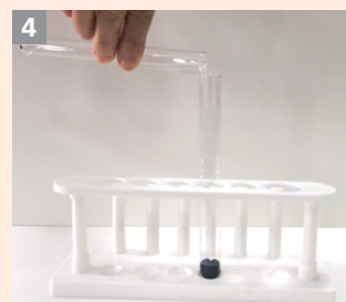
Reacția oxidului de cupru (II), CuO, cu acidul azotic, HNO 3
