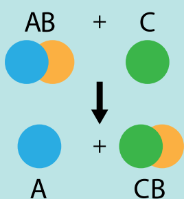
Reacția de substituție
