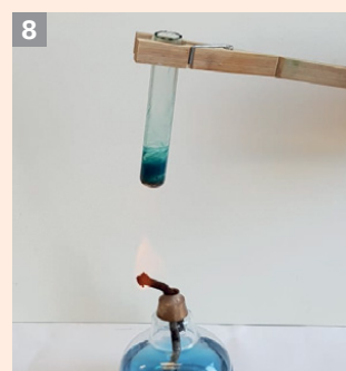
Descompunerea hidroxidului de cupru (II), \text{Cu(OH)}_2
