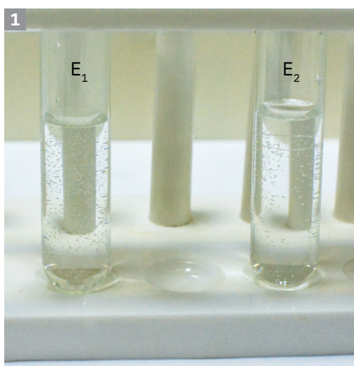
Eprubetele E_1 și E_2 cu apă oxigenată
