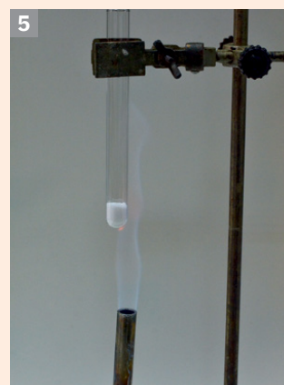
Încălzirea cloratului de potasiu, \text{KClO}_3
