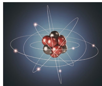
Atomul de carbon
