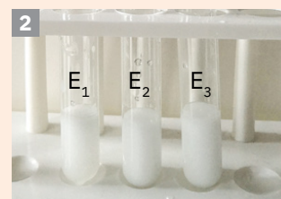
Formarea clorurii de argint, AgCl
