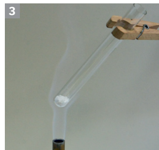
Descompunerea carbonatului de calciu
