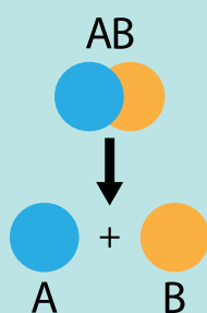
Reacția de descompunere
