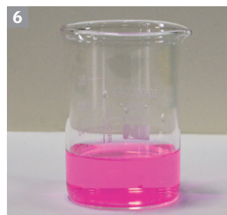
Colorarea soluției de fenolftaleină
