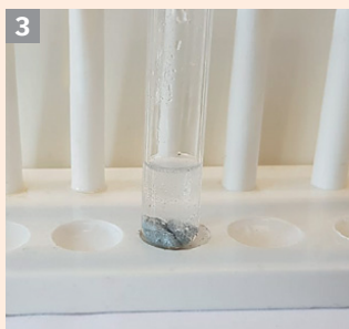
Reacția zincului cu acidul clorhidric
