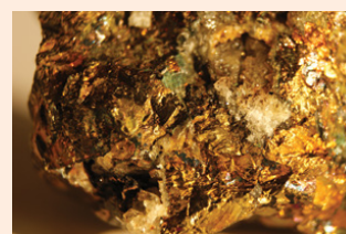
Minereul de pirită, \text{FeS}_2
