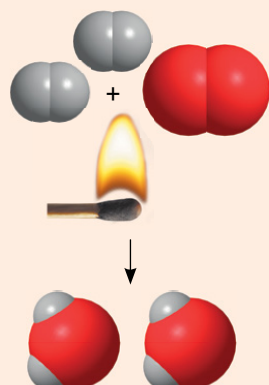
Arderea hidrogenului
