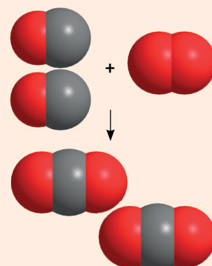
Obținerea dioxidului de carbon, \text{CO}_2
