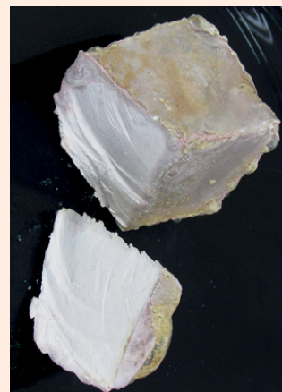
Sodiu metalic
