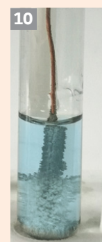
Depunerea argintului pe sârma de cupru și schimbarea culorii soluției în verde-albăstrui
