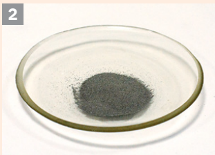
Pilitură de fier
