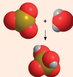
Obținerea acidului sulfuric, \text{H}_2\text{SO}_4
