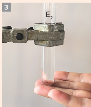
Reacția hidroxidului de potasiu, KOH, cu acidul azotic, HNO_3
