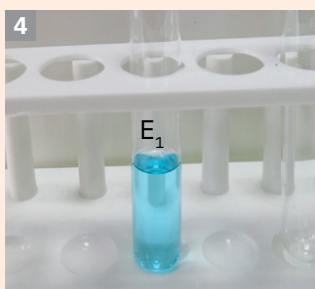
Soluție de sulfat de cupru rezultată în urma reacției
