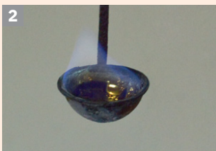
Arderea sulfului
