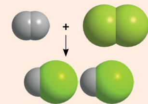
Obținerea acidului clorhidric, \text{HCl}
