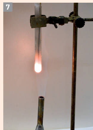
Evidențierea oxigenului format
