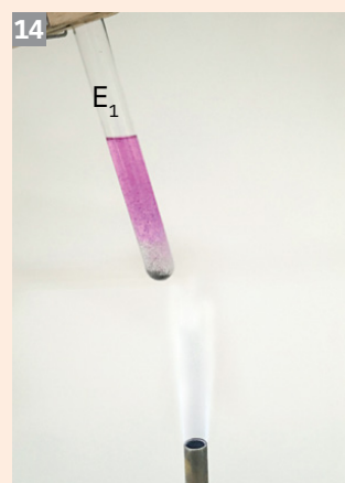
Reacția magneziului cu apa, în prezența soluției de fenolftaleină
